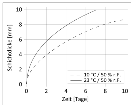
Diagramm 1: Durchhärtengeschwindigkeit Sikaflex®-527 AT
